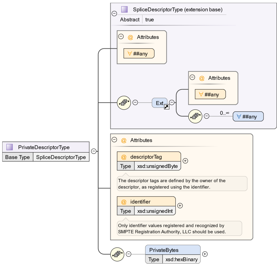
Figure 17 - PrivateDescriptorType
